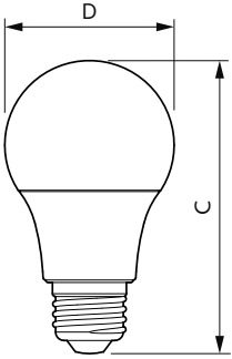
5A19/LED/930/FR/P/E26/ND/T20 6/1FB
